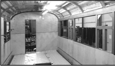
B 4229 mit geöffneter Setenwand
